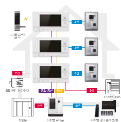
단독주택/아파트 설치구성도
